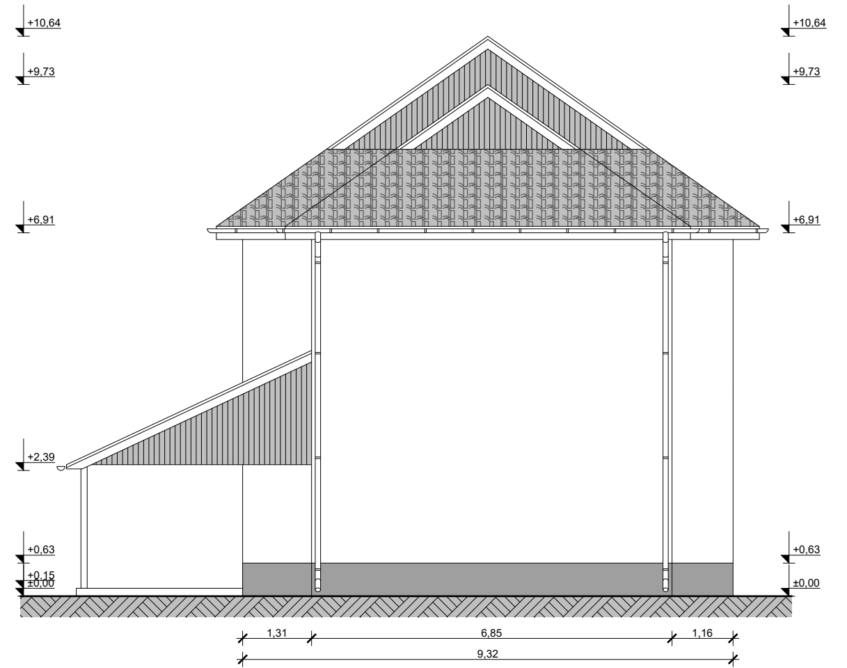
ÁLLAPOT ÉSZAKI HOMLOKZAT M=1:100
